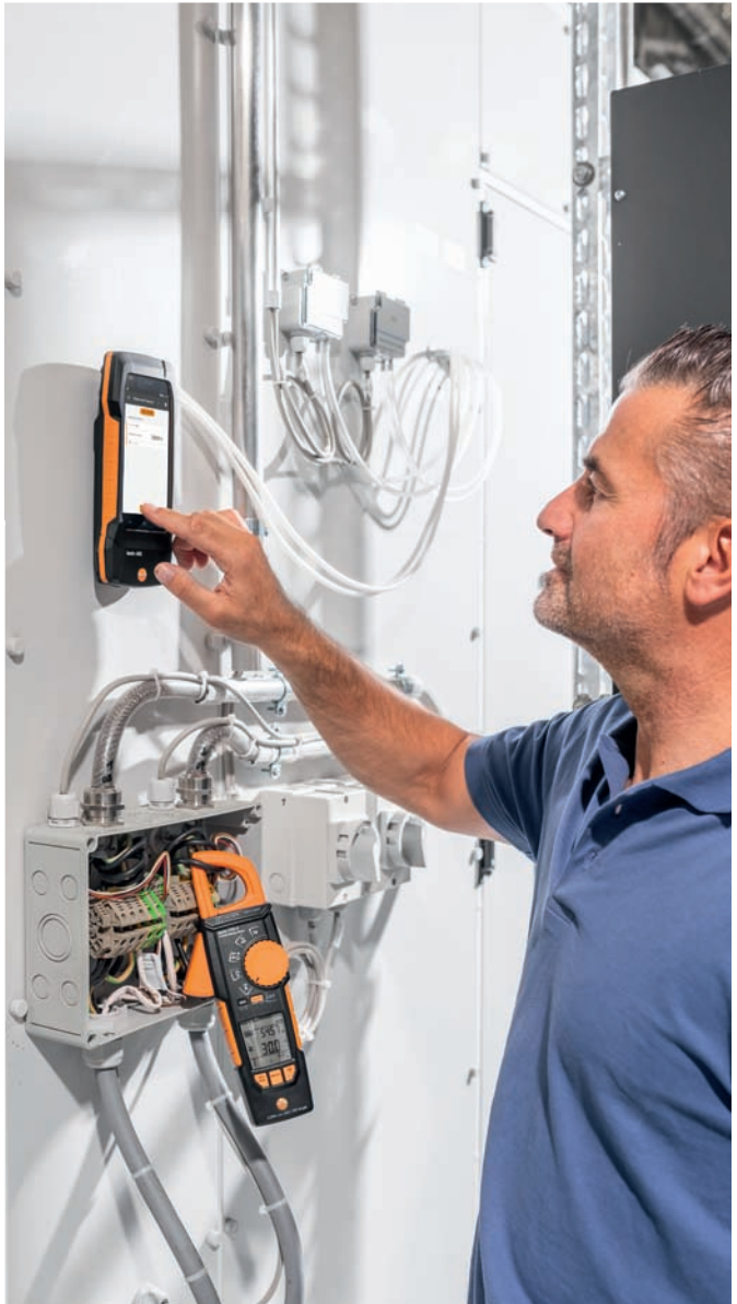
С testo 400 вы можете одновременно использовать до восьми зондов (4 с Bluetooth, 4 с кабелем)
